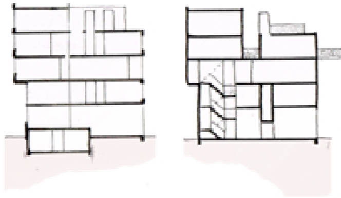
SECCION
