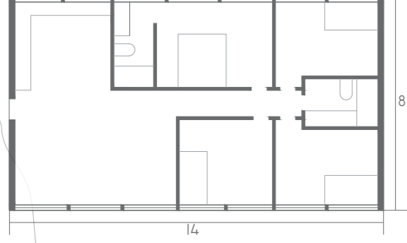
TIPOLOGIA APARTAMENTO
