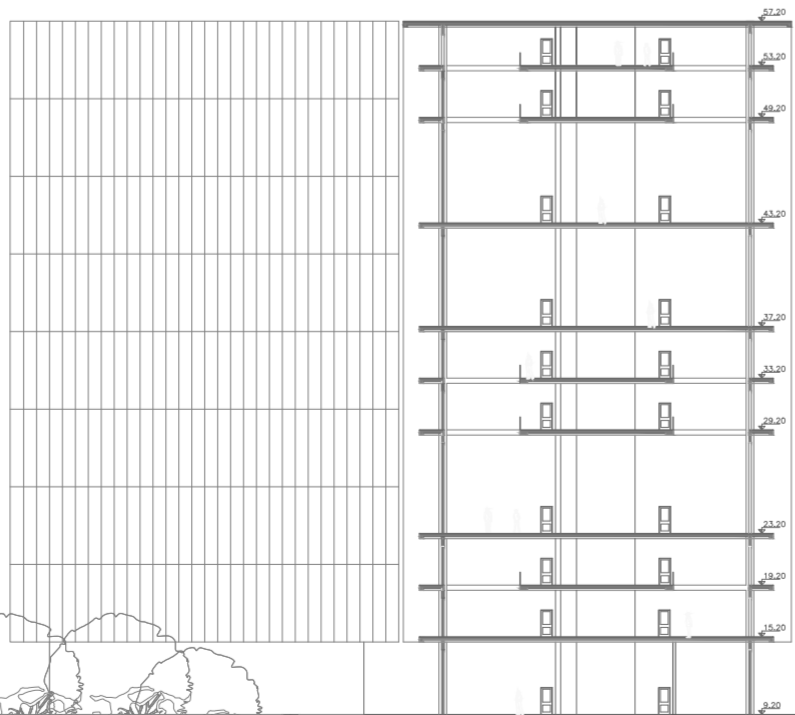
SECCIÓN A-A
