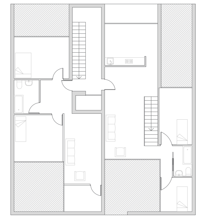
Planta baja tipo E 1:300
