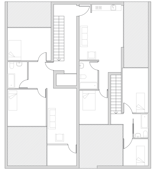
Planta alta tipo E 1:300
