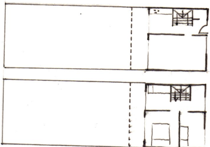
VIVIENDA UNIFAMILIAR
