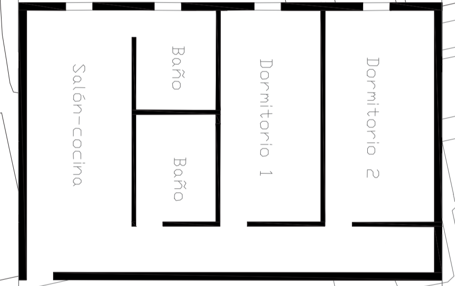
Tipología A (79 m 2 ) Vivienda con dos dormitorios E: 1/100
