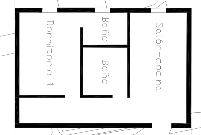
Tipología B (45 m 2 ) Vivienda con un dormitorio E: 1/100
