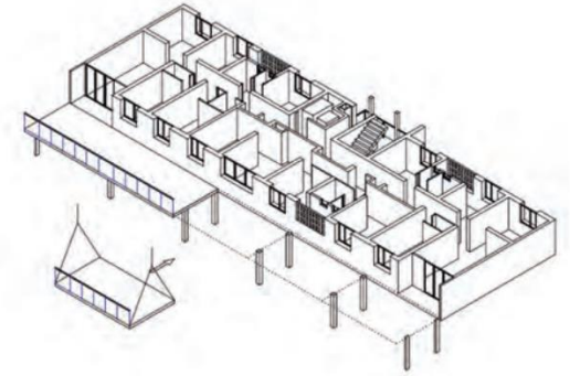
Montaje de los módulos de extensión
