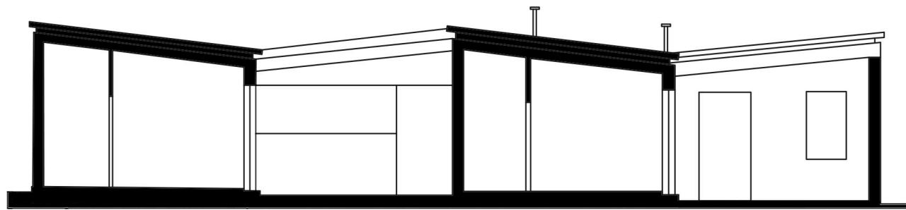
SECCIÓN B-B'
