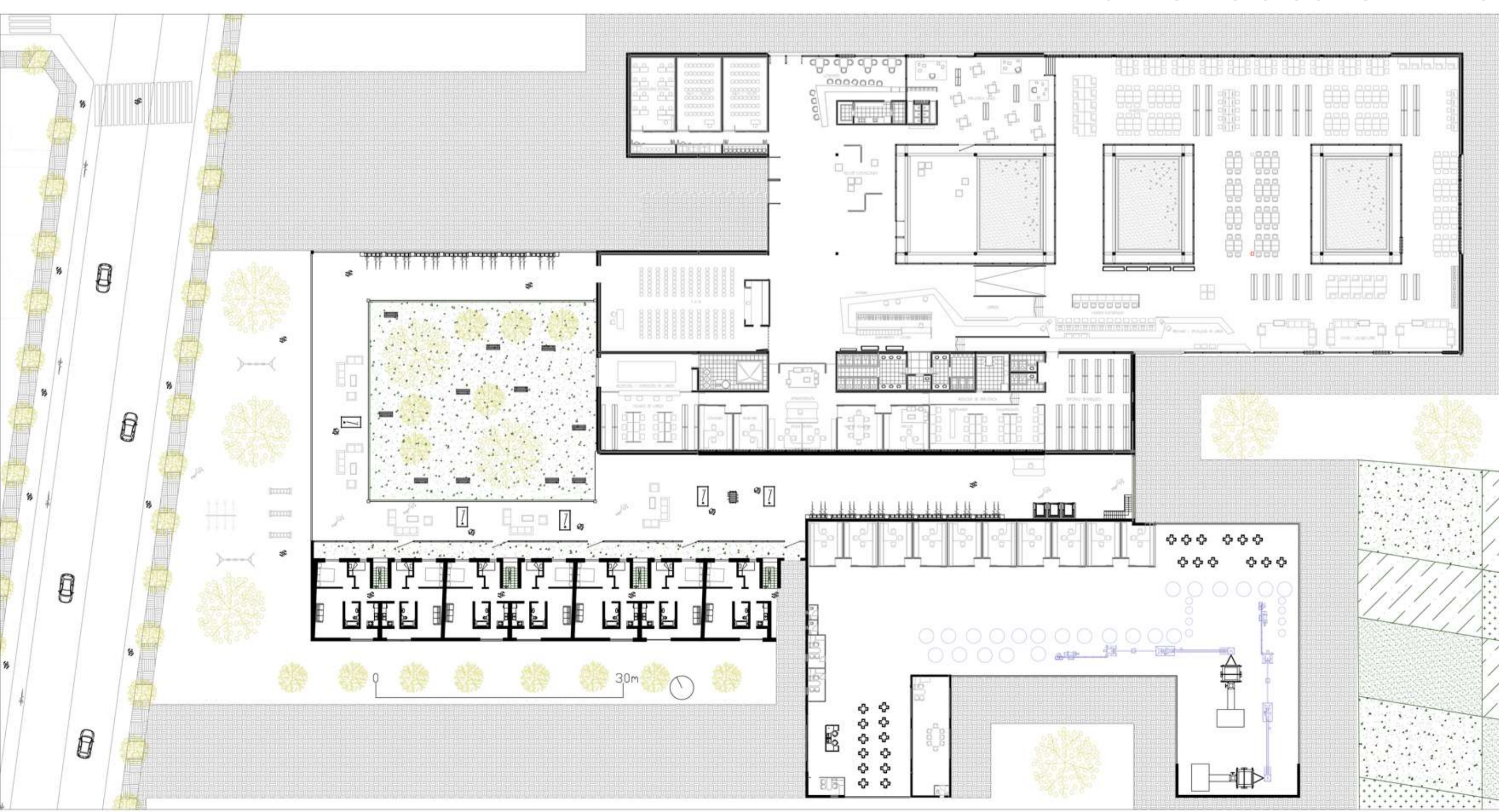
PLANTA BAJA-ESPACIO COMUNITARIO. 1ª PLANTA-8ª PLANTA. ESPACIO RESIDENCIAL.
