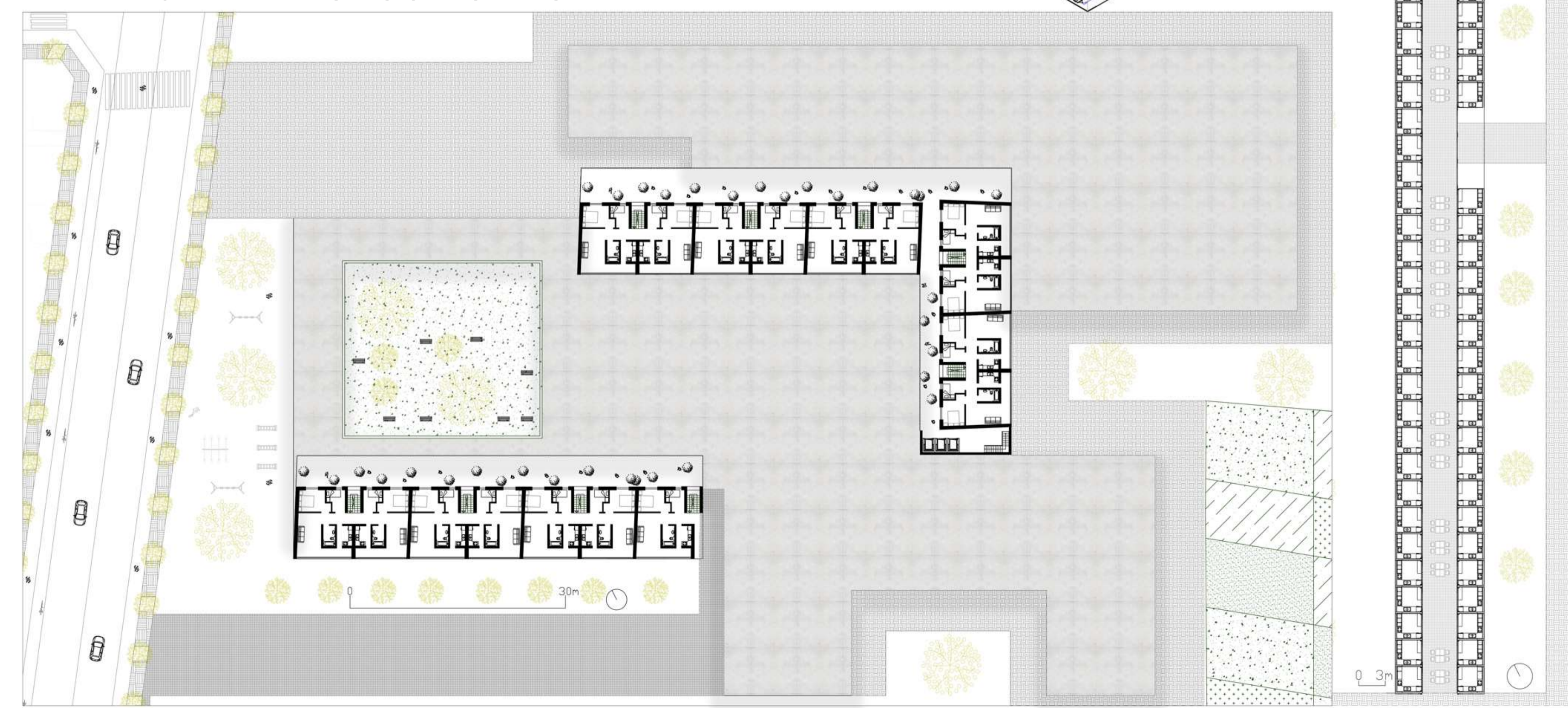
PLANTA BAJA-ESPACIO COMUNITARIO. 1ª PLANTA-8ª PLANTA. ESPACIO RESIDENCIAL.
