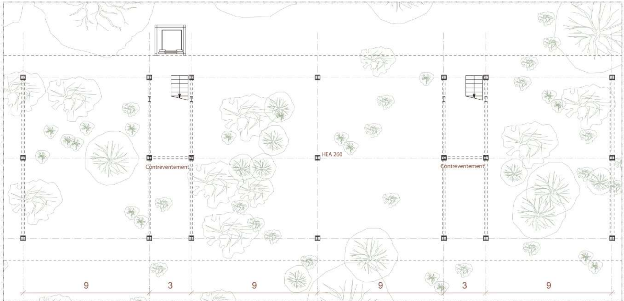
PLANTA
