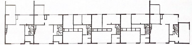
Plantas de la unidad residencial del vecindario de Vlashof.
