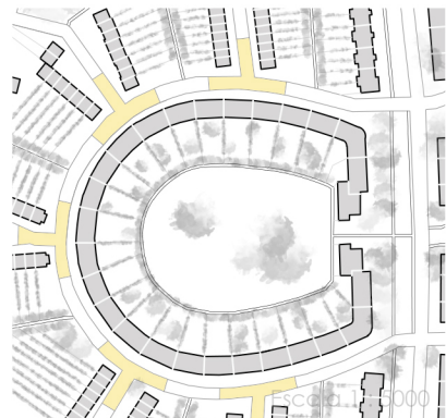
Edificios con entrante en un lado o en dos lados
