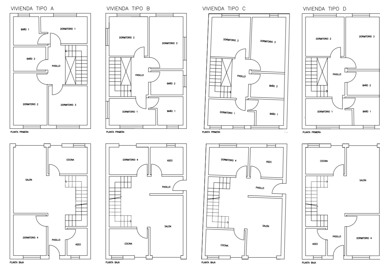
DENSIDAD 30 VIVIENDAS/HA
