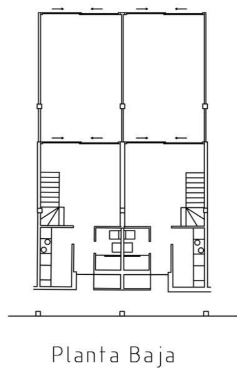
Casa Tipo Bloc con patio
