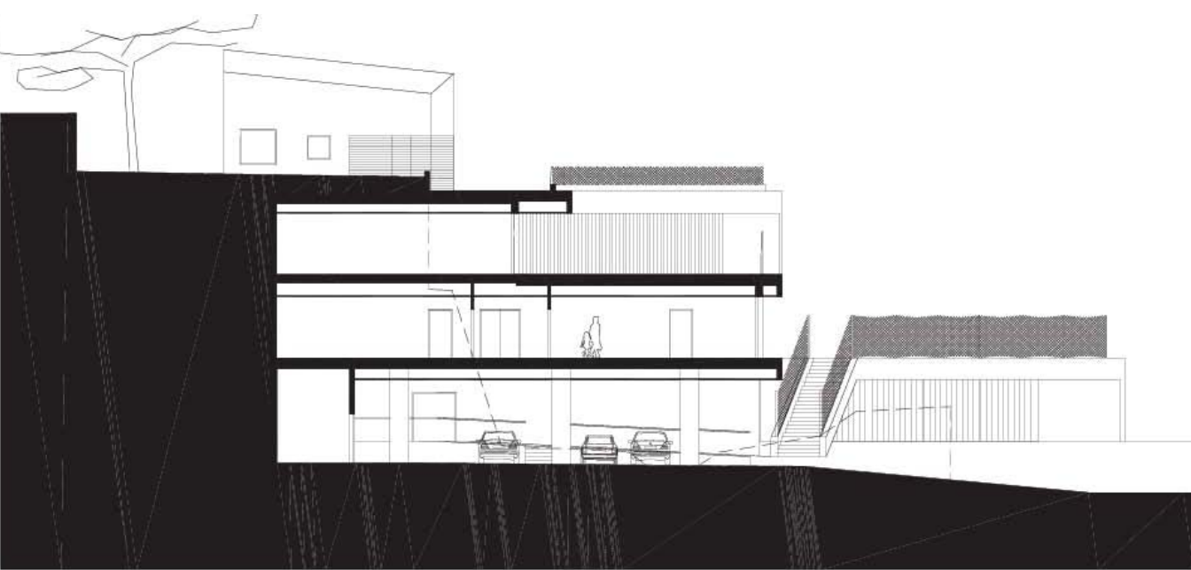
Sección
