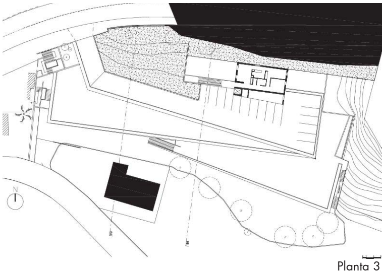
Planta 3
